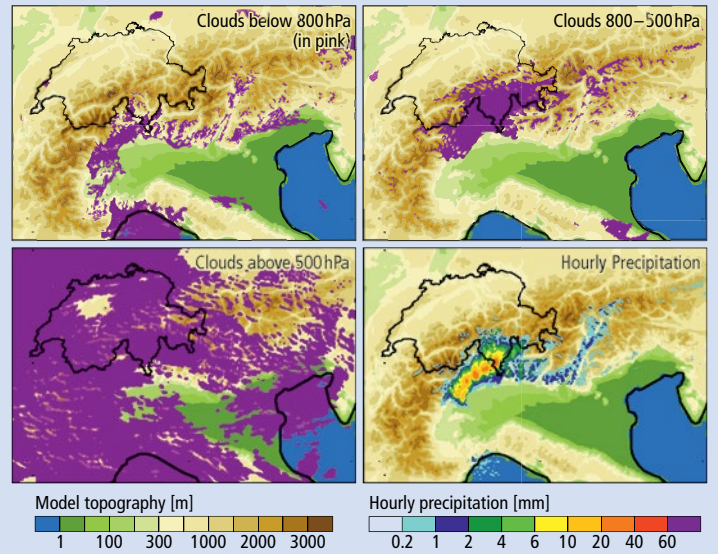
Fig. 47: Couverture nuageuse et précipitation horaire (en bas à droite) dans le modèle WRF sur une grille de 2 km pour le dimanche 27 septembre 1868 à 3 h. La couverture nuageuse en violet correspond aux basses couches (en haut à gauche), couches moyennes (en haut à droite) et hautes couches (en bas à gauche).
