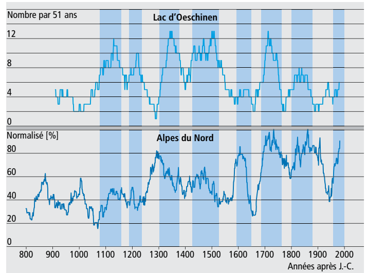
Fig. 65 : Fréquence des crues au cours des 1000 dernières années dans le lac d'Oeschinen 128 et dans les Alpes du Nord (valeur moyenne à partir de 10 lacs). 129
