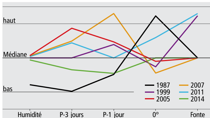
Fig. 22 : Prédiposition variable et déclenchement des plus grandes crues de la Kander (cf fig. 21). Humidité : saturation du sol au début de l'événement ; jours P-3, jour P-1 : quantité de précipitations en 3 et 1 jour(s) ; 0° : altitude de la limite du zéro degré ; fonte : contribution de la fonte des neiges.
