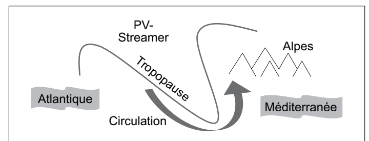
Fig. 7 : Situation météo pendant l'inondation de septembre 1993. En haut : tropopause (trait tillé en gars), hauteur de l'isobare 200 hPa (lignes continues), soulèvement des masses d'air (zones grises, en Pa/s) et vent (flèches) dans la haute troposphère. En bas : représentation schématique de la situation. 20
