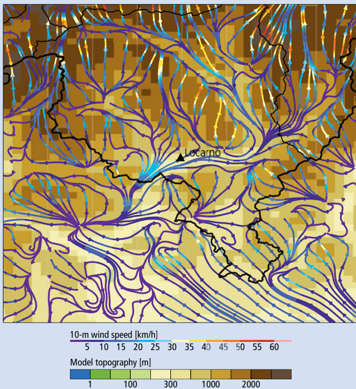
Fig. 46: Vent à 10 m du sol le dimanche 27 septembre 1868 à 12 h tel que reconstruit par le modèle WRF sur une grille de 2 km. La topographie du modèle est montrée en couleur, le vent par des flèches. La couleur des flèches représente la vitesse du vent. 32
