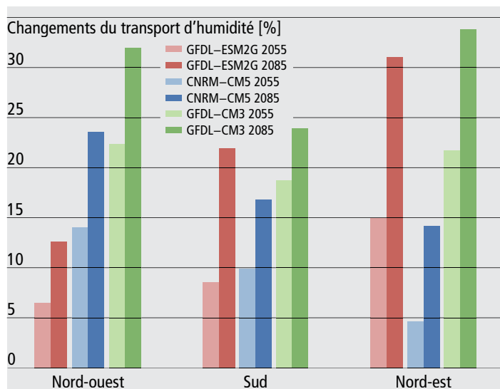
Fig. 11: Changements (en pourcents) de l'intensité des épisodes extrêmes de transport d'humidité pour le nord-est de la Suisse, le nord-ouest de la Suisse et le sud des Alpes, tels que calculés par trois modèles climatiques globaux différents. Les couleurs claires montrent les changements d'ici à la moitié du 21 ème siècle, les couleurs foncées d'ici à la fin du 21 ème siècle. Les trois modèles montrent une augmentation claire de l'intensité des épisodes extrêmes de transport d'humidité.
