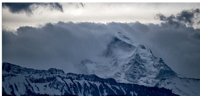
Fig. 13: Un « mur de Föhn » au-dessus de la Jungfrau. Le flux d'air venant du sud condense alors qu'il passe au-dessus des Alpes et un nuage se forme. Lorsque que l'air redescend de l'autre côté, le nuage s'évapore. Il en résulte un nuage stationnaire ressemblant à un mur.
