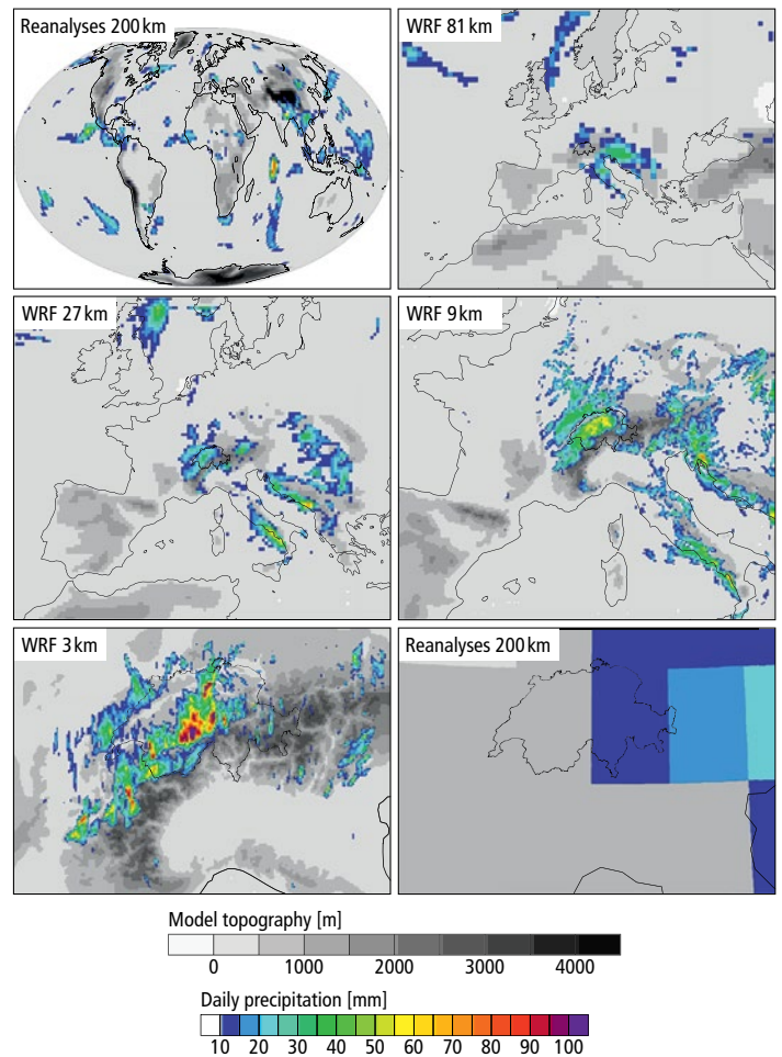
Fig. 45 : À partir de la réanalyse 20CR, des simulations WRF sont effectuées sur une grille de 81, 27, 9 et finalement 3 km de côté. Les précipitations journalières simulées pour le 22 août 2005 sont montrées. La réanalyse est aussi montrée en bas à droite pour le même domaine que la simulation WRF à 3 km, pour comparaison.
