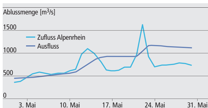
Abb. 19: Die dämpfende Wirkung des Bodensees bei den beiden Hochwasserereignissen im Mai 1999 (Daten: BAFU)
