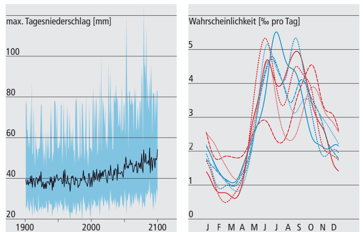
Abb. 75: Entwicklung der maximalen Tagesniederschläge pro Jahr für das Aare-Einzugsgebiet aus den CMIP5-Simulationen (dunkelblau: Mittelwert aller Simulationen, hellblau: Maxima und Minima) (links). Kalendertag des maximalen Tagesniederschlags eines Jahres in der Gegenwart (1971–2005, blau) und der Zukunft (rot, 2065–2099, unterschiedliche Strichsignaturen stellen unterschiedliche Modellensembles dar) (rechts). 148
