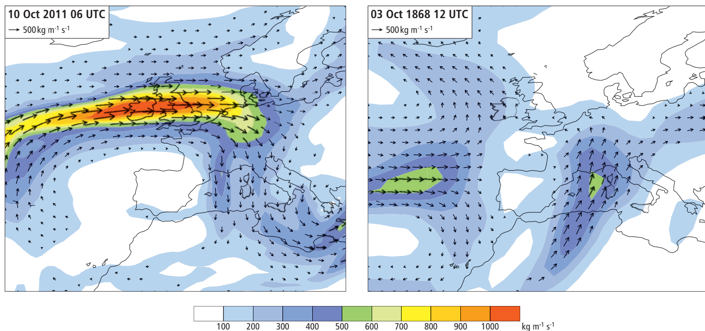
Abb. 10: Vertikal integrierter atmosphärischer Feuchtetransport ( \text{kg m}^{-1} \text{s}^{-1} , Farbschattierung) am 10. Oktober 2011 am Morgen (6 UTC, links) und 3. Oktober 1868 am Mittag (12 UTC, rechts). Die Pfeile zeigen die Transportrichtung. Der atmosphärische Fluss ist links als lange, schmale Struktur über dem Atlantik erkennbar. Im Oktober 2011 erreichte die feuchte Luft die Alpen von Norden, am 3. Oktober 1868 aus Süden. 25
