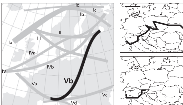
Abb. 6: Links: Klassifikation der Zugbahnen von Tiefdruckgebieten zwischen 1876 und 1880 17 nach W. J. van Bebber. 16 Rechts: Zugbahnen der Tiefdruckgebiete während der Hochwasserereignisse vom 10. bis 13. August 2002 (oben) und vom 20. bis 24. August 2005 (unten). 18
