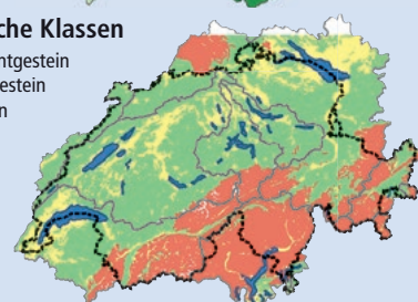
Abb. 20: Faktoren der Grunddisposition im Schweizer Vergleich. Anteile von Geländeneigung von 15% (oben) und wasserableitende, kristalline Geologie (unten), steht einem hohen Waldanteil gegenüber (Mitte).
