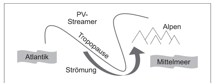
Abb. 7: Wetterlage während des Hochwasserereignisses vom September 1993. Oben: Tropopause (fett gestrichelt), geopotenzielle Höhe (auf 200hPa; durchgezogene Linien), Hebung der Luftmassen (Grauschattierung; Pals) und Wind (Pfeile) in der oberen Troposphäre. Unten: Entsprechendes Konzept der Anströmung. 20
