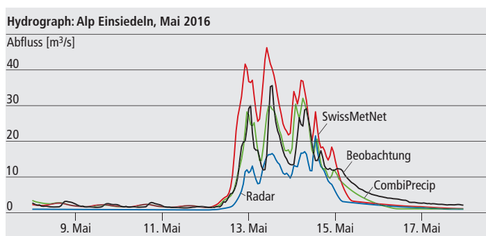
Abb. 37: Abflusssimulation der Alp bei Einsiedeln [ m^3 s^{-1} ] mit dem hydrologischen Modell PREVAH für die Periode vom 8. bis 17. Mai 2016. Drei Regenprodukte wurden für die Simulationen verwendet: interpolierte SwissMetNet-Daten (rot), Radardaten (blau) und das CombiPrecip Produkt (grün).
