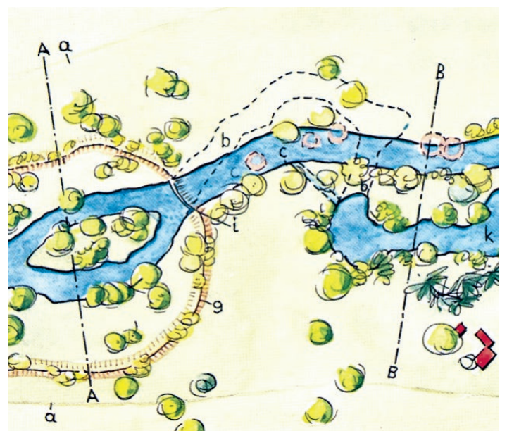
Abb. 63: Die Darstellung des engen Sporensystems, das im 19. Jahrhundert unter anderem an der Rhone angewendet wurde (Bild links), und des Konzepts «Mehr Raum den Fliessgewässern» aus der Wegleitung «Hochwasserschutz an Fliessgewässern» von 1982 (Bild rechts) zeigen deutlich den Wandel des Hochwasserschutzes vom 19. Jahrhundert bis heute.
