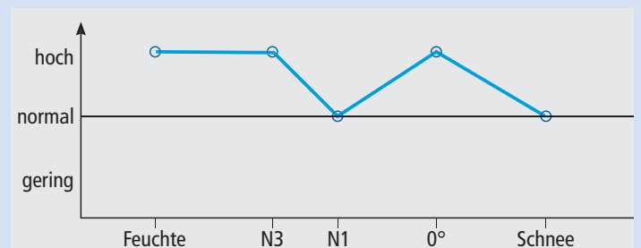
Abb. 26: Schematische Darstellung des Einflusses der Faktoren (Beschreibung vgl. Abb. 22) der variablen Disposition auf das Hochwasserereignis von 1868.
