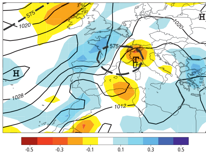
Abb. 8: Wetterlage während des Hochwasserereignisses am 21. August 2005. 25 Unter einem Kaltlufttropfen auf 500hPa (ca. 5km, fett gestrichelt 12 ) entwickelt sich ein Genuatief (T); durchgezogene Linien markieren den Luftdruck am Boden in hPa, das zwischen zwei Hochdruckgebieten (H) blockiert ist. Farblich schattiert ist die Vertikalbewegung (Pa/s; rot bedeutet Hebung) in ca. 5km Höhe (500hPa).
