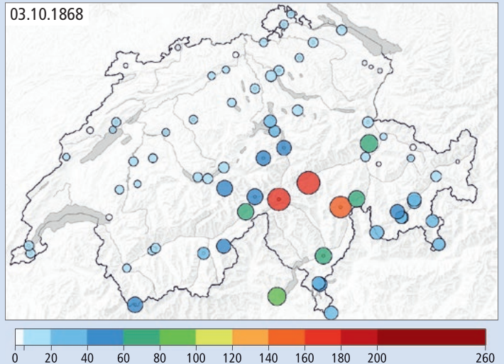
Abb. 33: Messungen der täglichen Niederschlagssumme (Millimeter oder Liter pro Quadratmeter innerhalb von 24 Stunden) in der Schweiz am 3. Oktober 1868. 12,32
