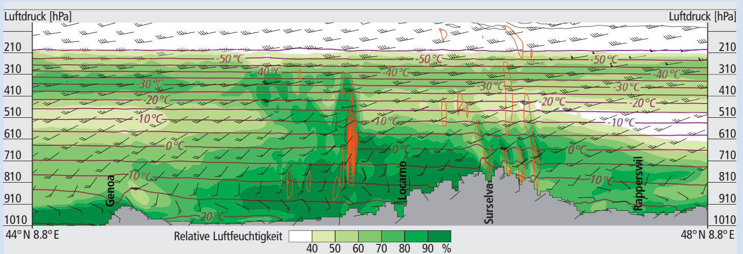
Abb. 16: Querschnitt durch die Alpen am 26. September 1868 am Abend (21 UTC) von Süden (links) nach Norden (rechts). Die Daten stammen aus einer Simulation mit dem Wettermodell WRF (vgl. S. 26) in 2 km Auflösung und 40 Schichten. Die Topographie (dunkelgraue Fläche) entspricht der Modelltopographie. Farben zeigen die relative Luftfeuchtigkeit an. Windspitzen zeigen den horizontalen Wind an: nach oben für Südwind (Wind aus Süden), nach rechts für Westwind usw. Je mehr Seitenbalken die Windspitzen haben, desto stärker ist der Wind (10 Knoten, also etwa 20 km/h pro Balken). Die orangen Konturen stellen Bereiche aufsteigender Luft dar. Die Temperatur wird durch rotviolette Linien mit Beschriftung angezeigt. Die Nullgradgrenze liegt bei ca. 630 hPa (ca. 4000 m ü.M.).
