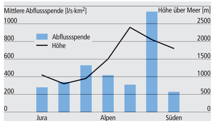
Abb. 18: Die Abflussspende eines Hochwassers mittlerer Grösse entlang eines Nord-Süd-Profiles durch die Schweiz. 37
