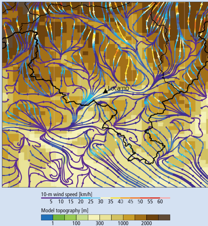
Abb. 46: Der Wind in 10m Höhe über dem Tessin am Sonntag, 27. September 1868 am Mittag (12 UTC), rekonstruiert durch das WRF-Modell mit einer Rasterweite von 2km. Die Topographie des Modells wird durch die Farbe, der Wind durch Pfeile dargestellt (Pfeilfarben stellen die Windgeschwindigkeit dar). 32
