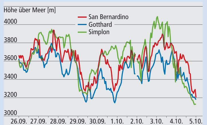
Abb. 25: Die mittels regionalen Wettermodells (vgl. S. 26) rekonstruierte Nullgradgrenze an drei ausgewählten Standorten 1 zeigt die hohe Nullgradgrenze von Ende September bis Anfang Oktober 1868. 32
