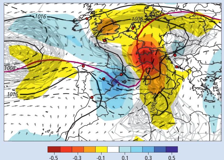
Abb. 44: Reduzierter Bodendruck (hPa; durchgezogene schwarze Linien; graue Pfeile für das Ensemble), Wind auf 850hPa (1,5 km Höhe; graue Pfeile), Druck auf 500 hPa (ca. 5 km Höhe; gestrichelte schwarze Linien), vertikale Bewegung der Luftmassen auf 500 hPa (negativ bedeutet Hebung) und Tropopause (1,5 PVU; rote Linie) aus 20CR für den 22. September 1868 am Mittag (12 UTC). Die eingeflossenen Messungen sind als rote Punkte markiert.
