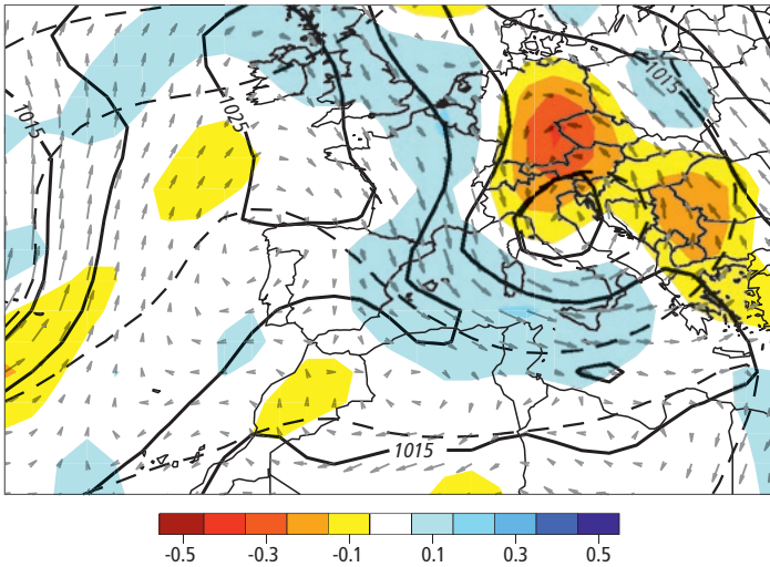
Abb. 42: Wetterkarte aus der 20CR-Reanalyse 25 für den 14. Juni 1910 Mittag (12 UTC): reduzierter Bodendruck (hPa; fette schwarze Linien), Windfeld auf 850hPa (ca. 1,5 km Höhe; graue Pfeile), Druck auf 500 hPa (ca. 5 km Höhe; fette gestrichelte Linien), vertikale Bewegung der Luftmassen auf 500 hPa (negativ bedeutet Hebung).
