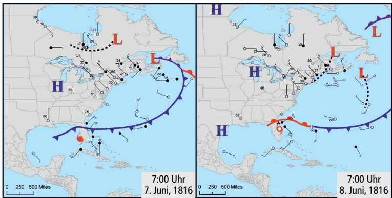
Abb. 12. Wetterkarten für den 7. und 8. Juni 1816 sowie Beobachtungen von Wind, Temperatur (°F), Bewölkung (offene/gefüllte Kreise) und Niederschlag (Symbole neben den Windpfeilen), basierend auf einer Zusammenstellung von Beobachtungen von Mike Chenoweth (2009). 99
